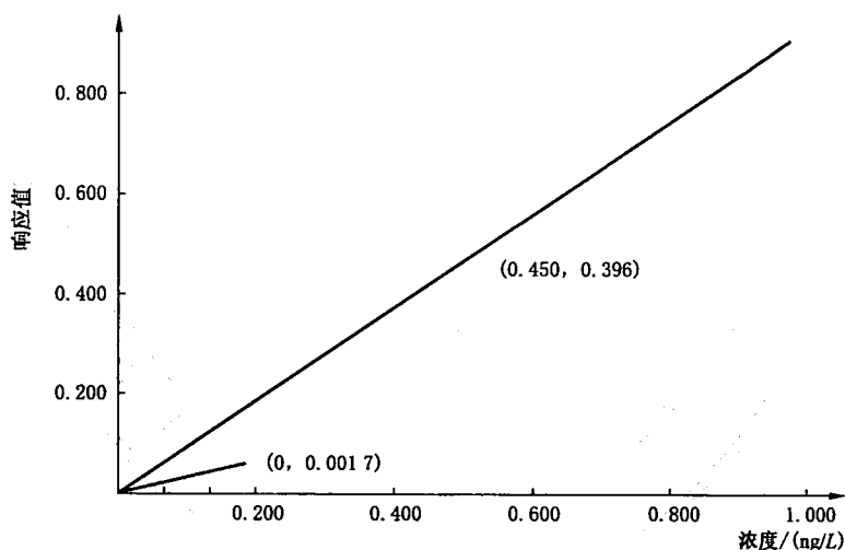
图 1 校准曲线
