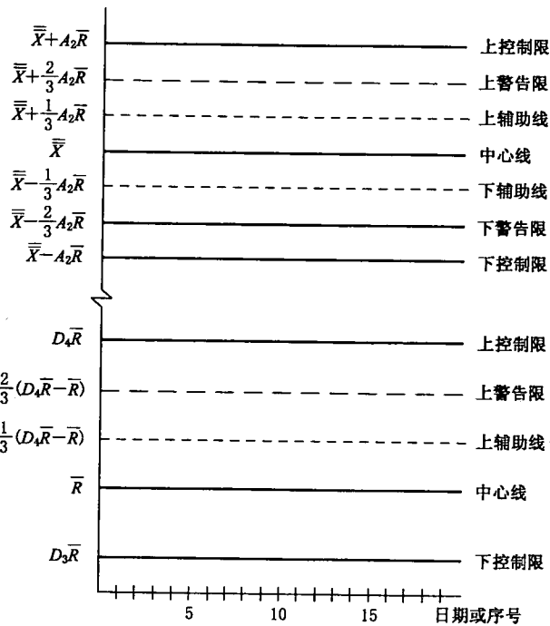
图5 均数-极差控制( \bar{X}-R )图基本组成
