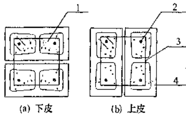
图 9.4.13 配筋砌块砌体柱截面示意
