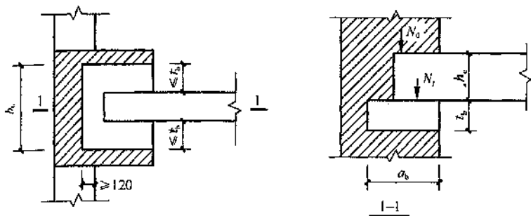
图 5.2.5 壁柱上设有垫块时梁端局部受压
