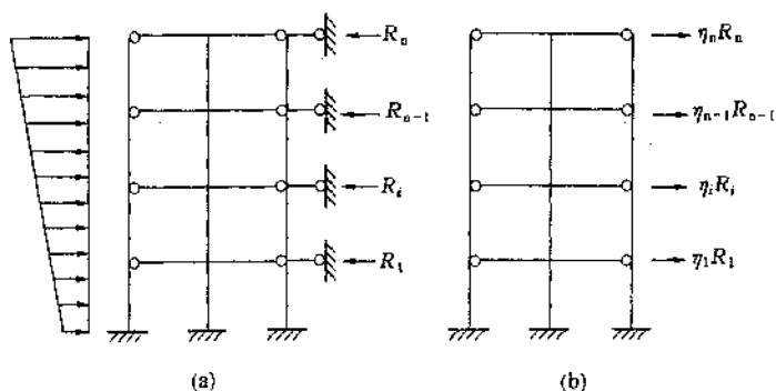
图 C.0.1 刚弹性方案房屋的静力计算简图
