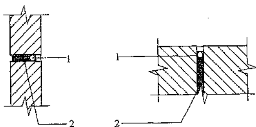
图 6.5.7 控制缝构造
