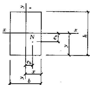
图 D. 0. 3 双向偏心受压
