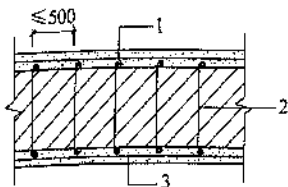
图 8.2.6 混凝土或砂浆 面层组合墙
