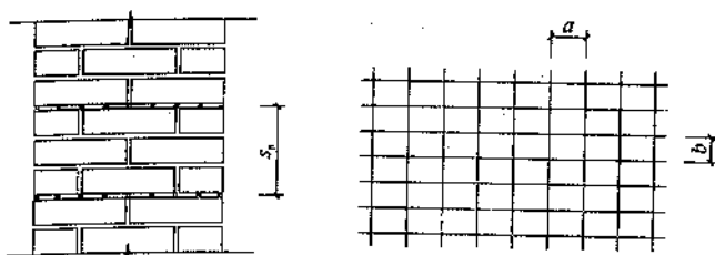
图 8.1.2 网状配筋砖砌体
