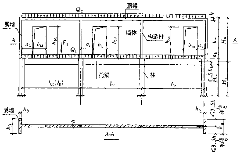
图 7.3.3 墙梁计算简图
