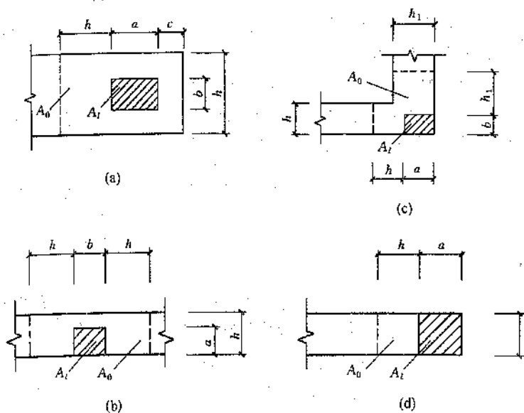
图 5.2.2 影响局部抗压强度的面积 A_0
