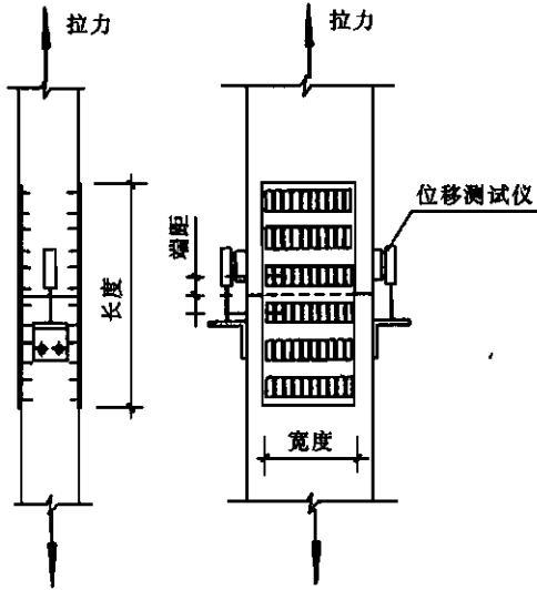
图 M. 2. 2a 荷载平行于木纹及齿板主轴 \alpha=0^\circ \quad \theta=0^\circ
