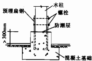
图 7.6.5 木柱与基础锚固和 柱脚防潮
