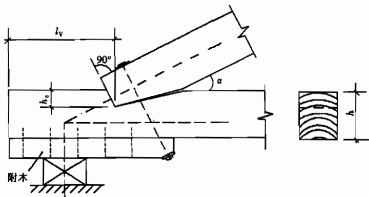
图 6.1.1-1 单齿连接
