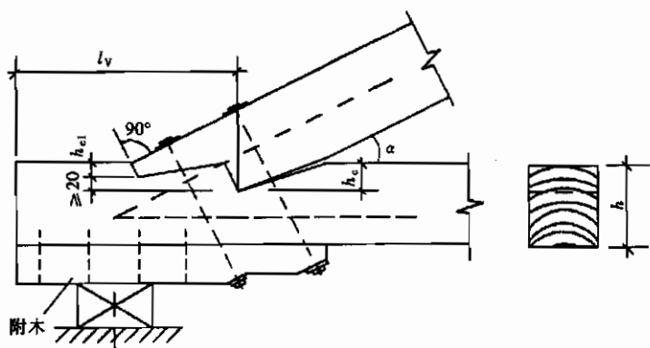
图 6.1.1-2 双齿连接
