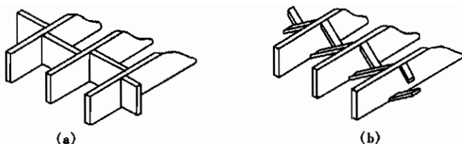
图 9.3.6 搁栅间支撑示意图
