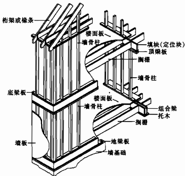
图 7 轻型木结构基本构造示意图
