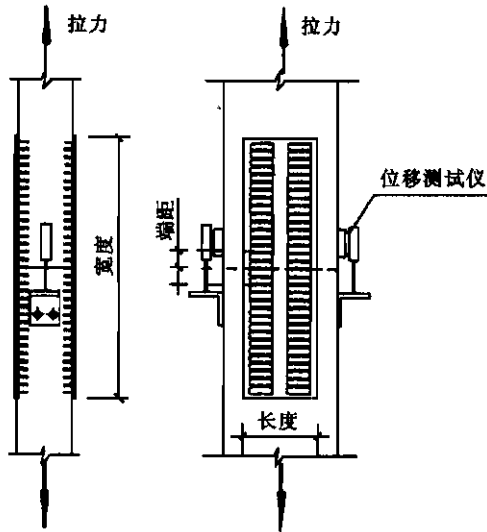
图 M. 2. 2b 荷载平行于木纹但垂直于齿板主轴 \alpha=0^\circ \quad \theta=90^\circ
