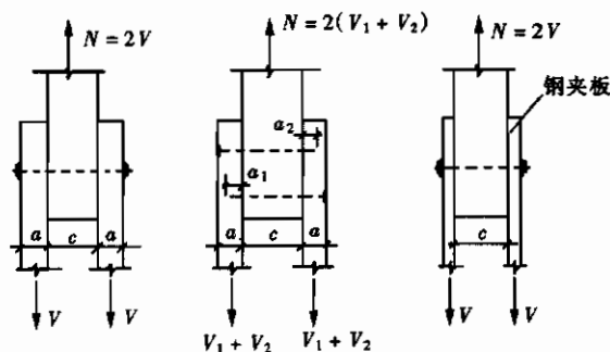
图 6.2.1-1 双剪连接
