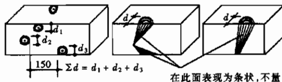
附图 A.1 木节量法
