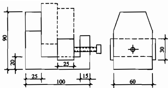
图 E.4 胶缝剪切试验装置
