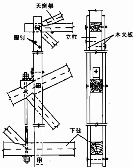
图 7.4.1 立柱的木夹板示意图
