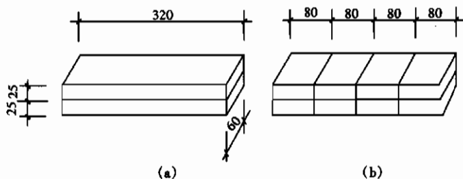
图 E. 3. 1 试条的尺寸
