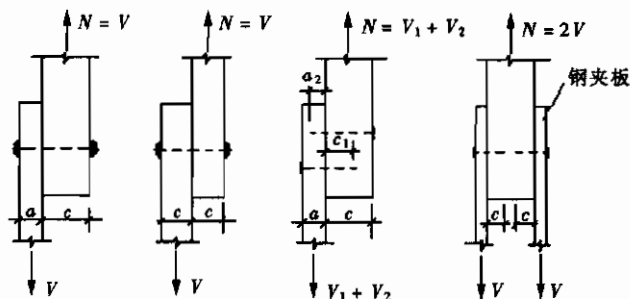
图 6.2.1-2 单剪连接
