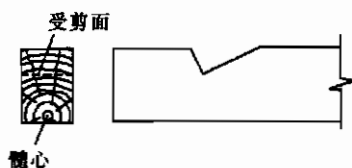
图 7.3.4 受剪面避开髓心示意图
