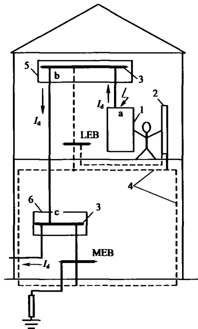
图3 局部等电位联结的作用
