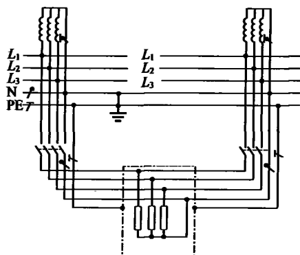
图 2 在 TN-S 系统中,采用具有断开中性极的开关可避免产生杂散电流
