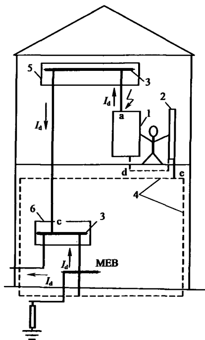
图4 辅助等电位联结的作用
