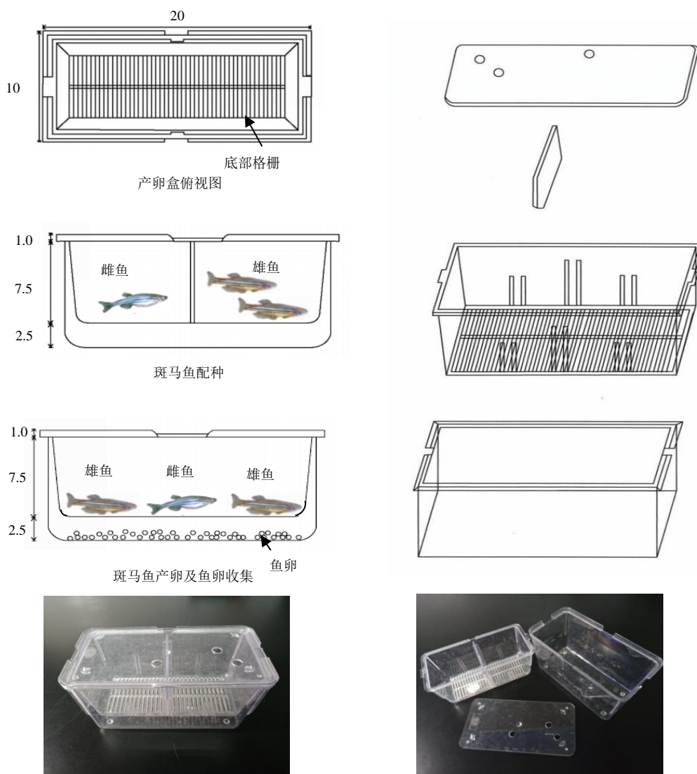
图 4 产卵盒示意图（单位：cm）
