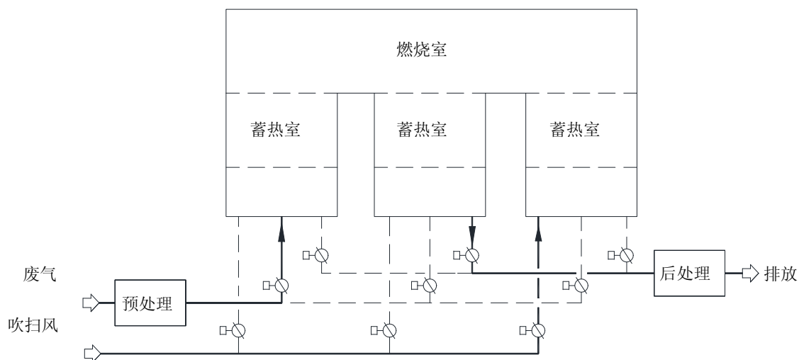
图2 固定三室蓄热燃烧工艺流程示意图
