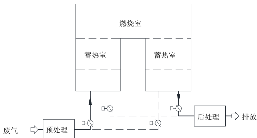
图1 固定两室蓄热燃烧工艺流程示意图
