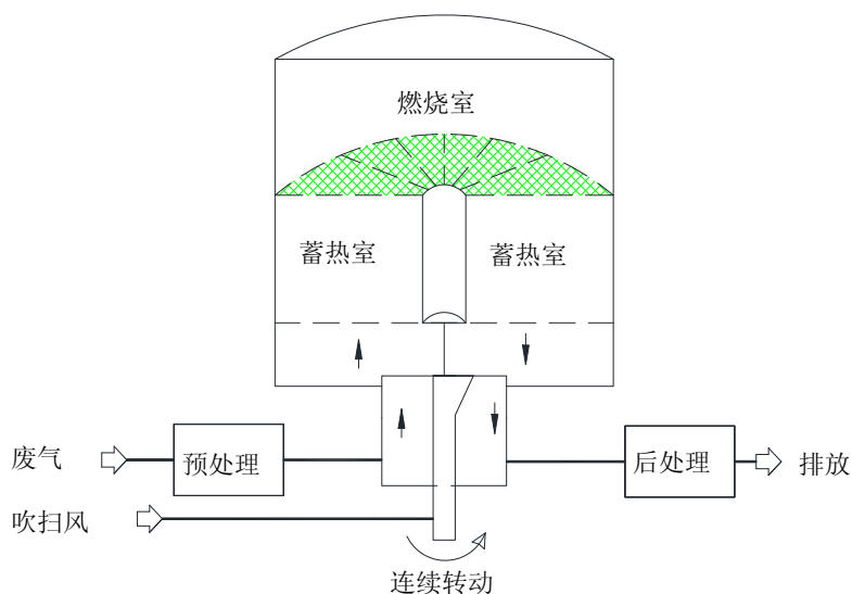
图3 旋转式蓄热燃烧工艺流程示意图
