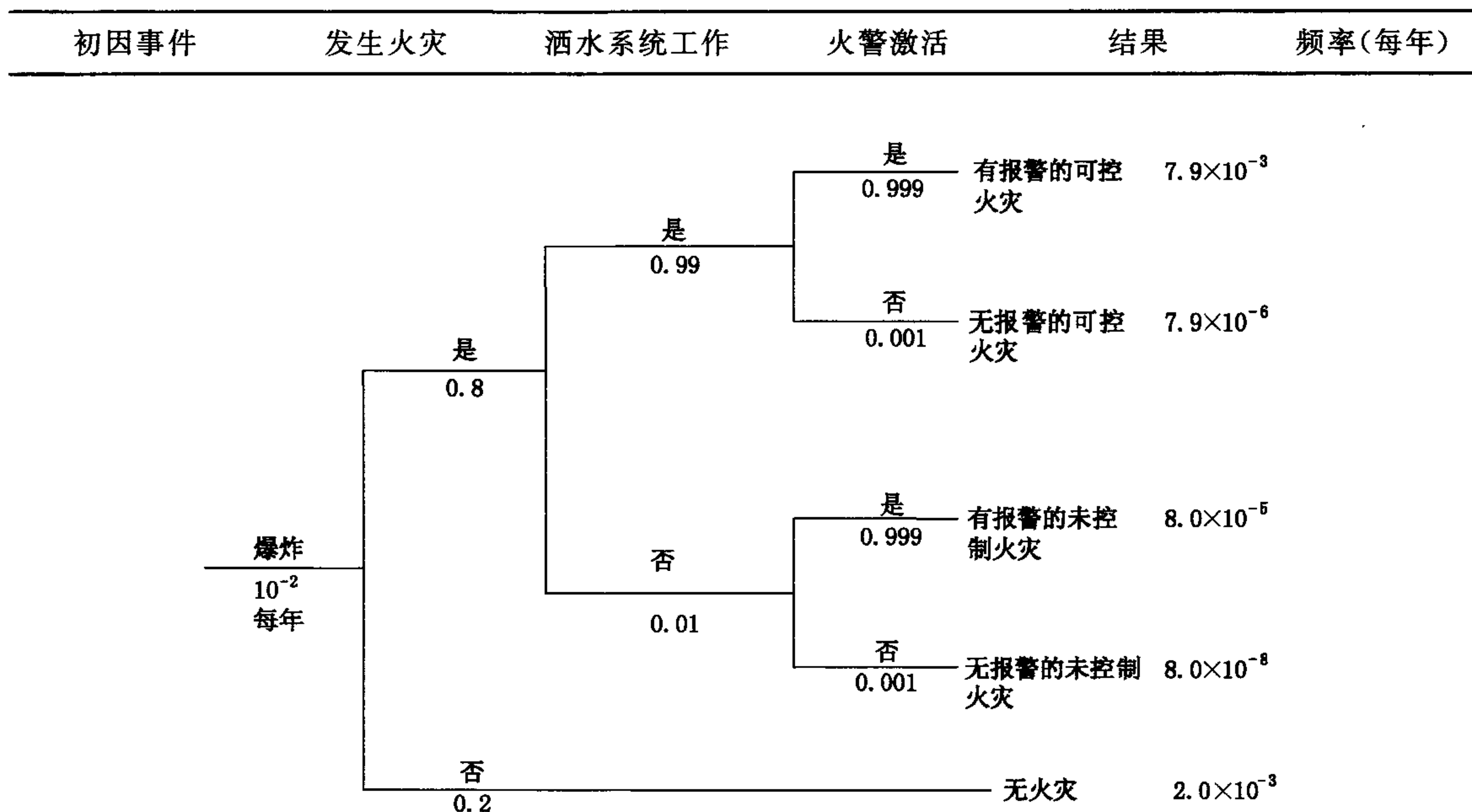
图 B. 4 事件树示例
