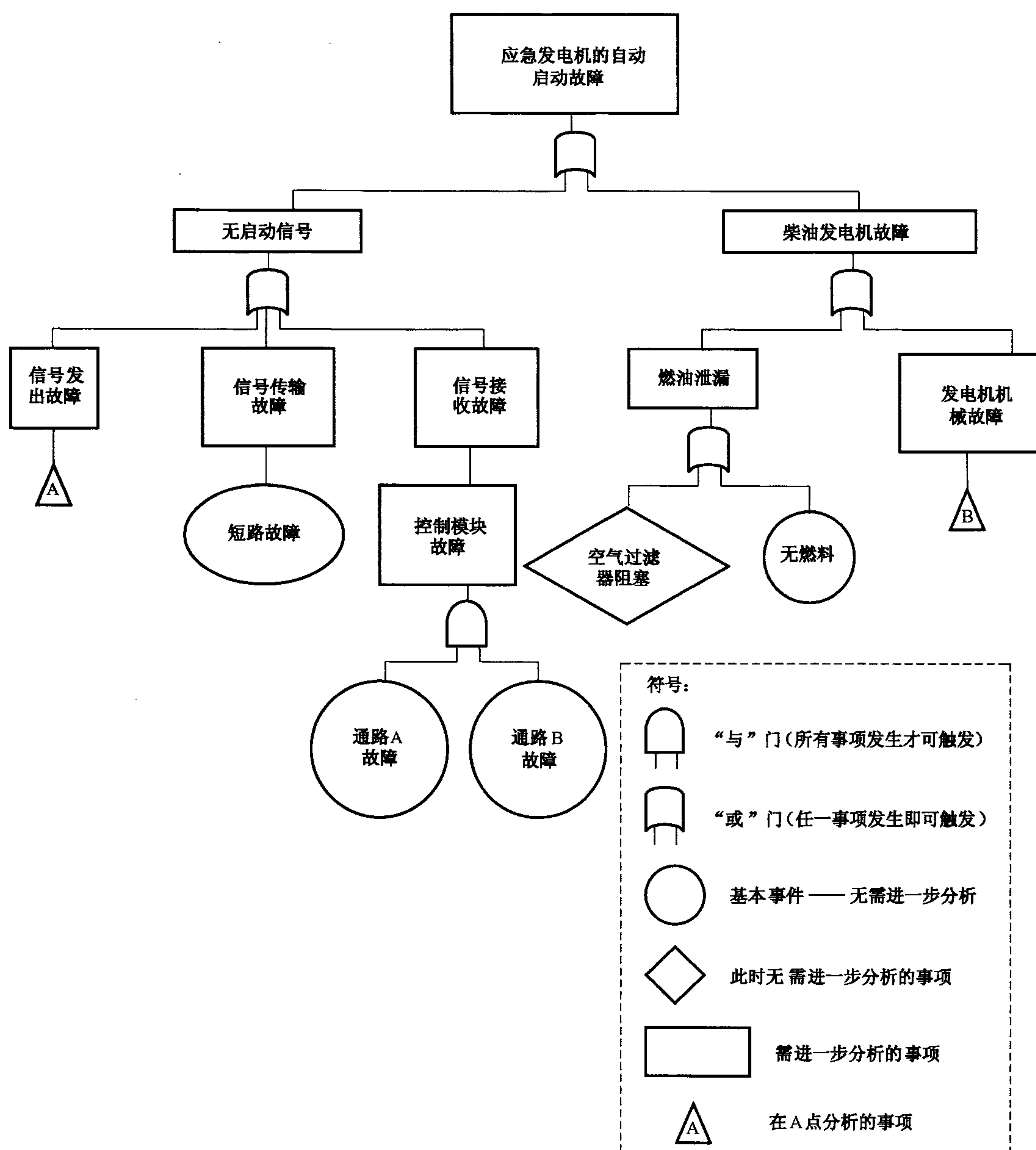
图 B.3 FTA 示例
