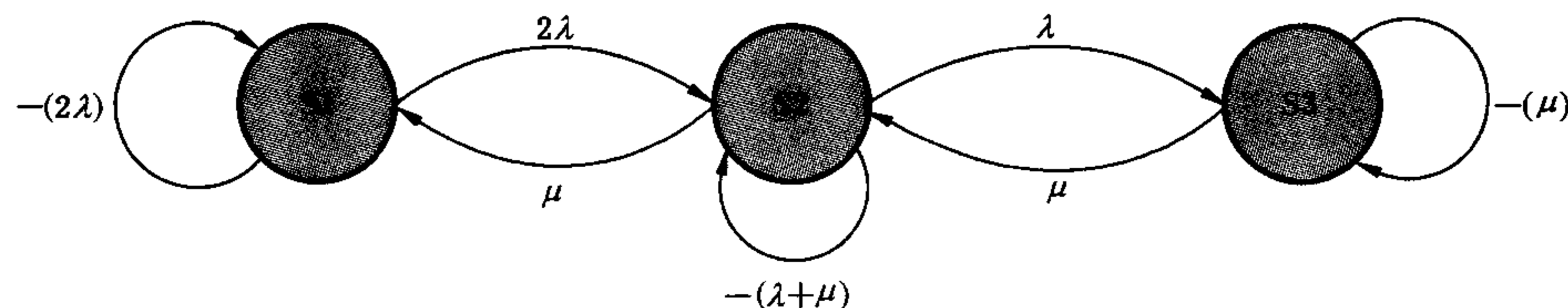
图 B.8 状态转移图
