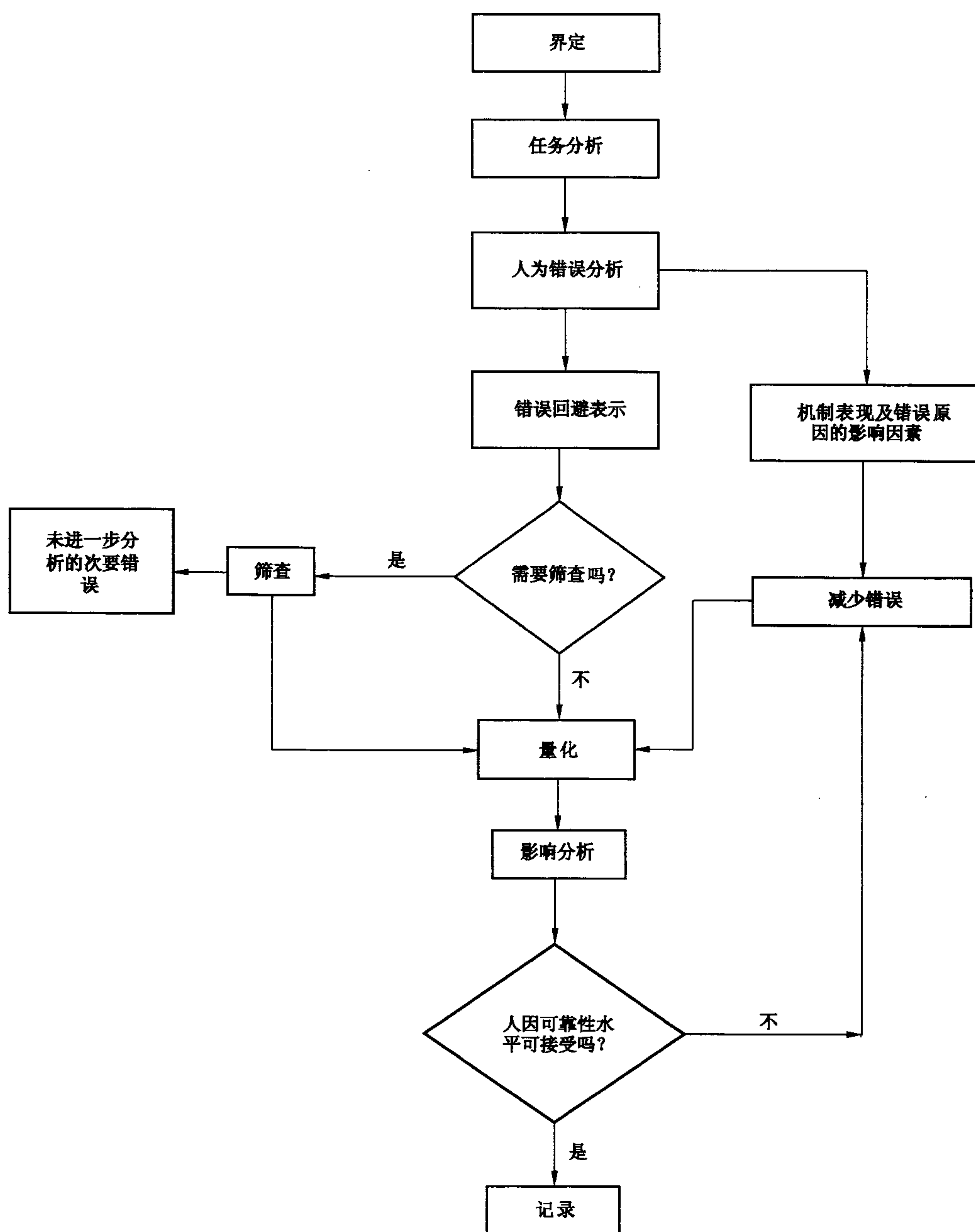
图 B.2 人因可靠性分析
