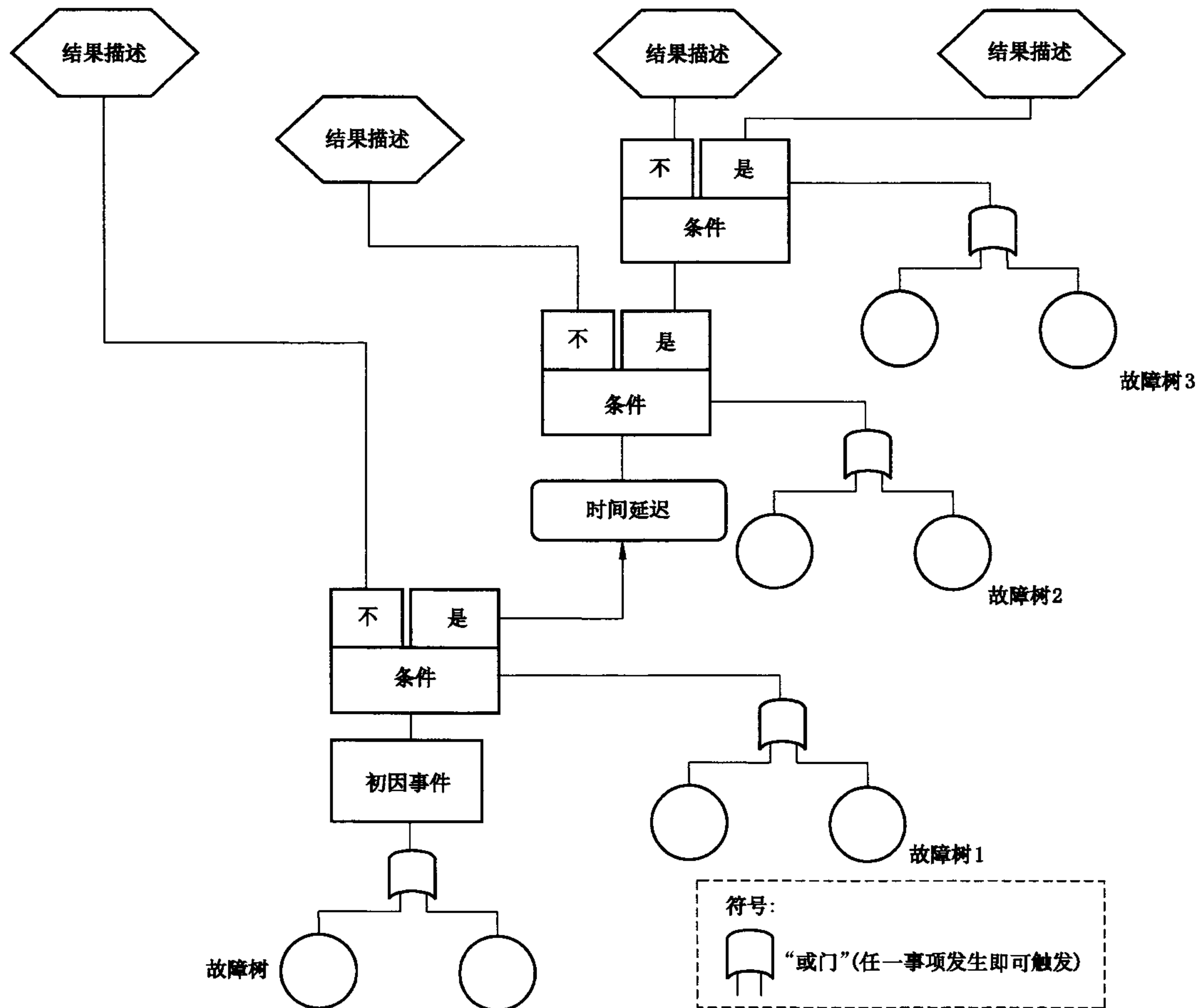
图 B. 5 因果分析示例
