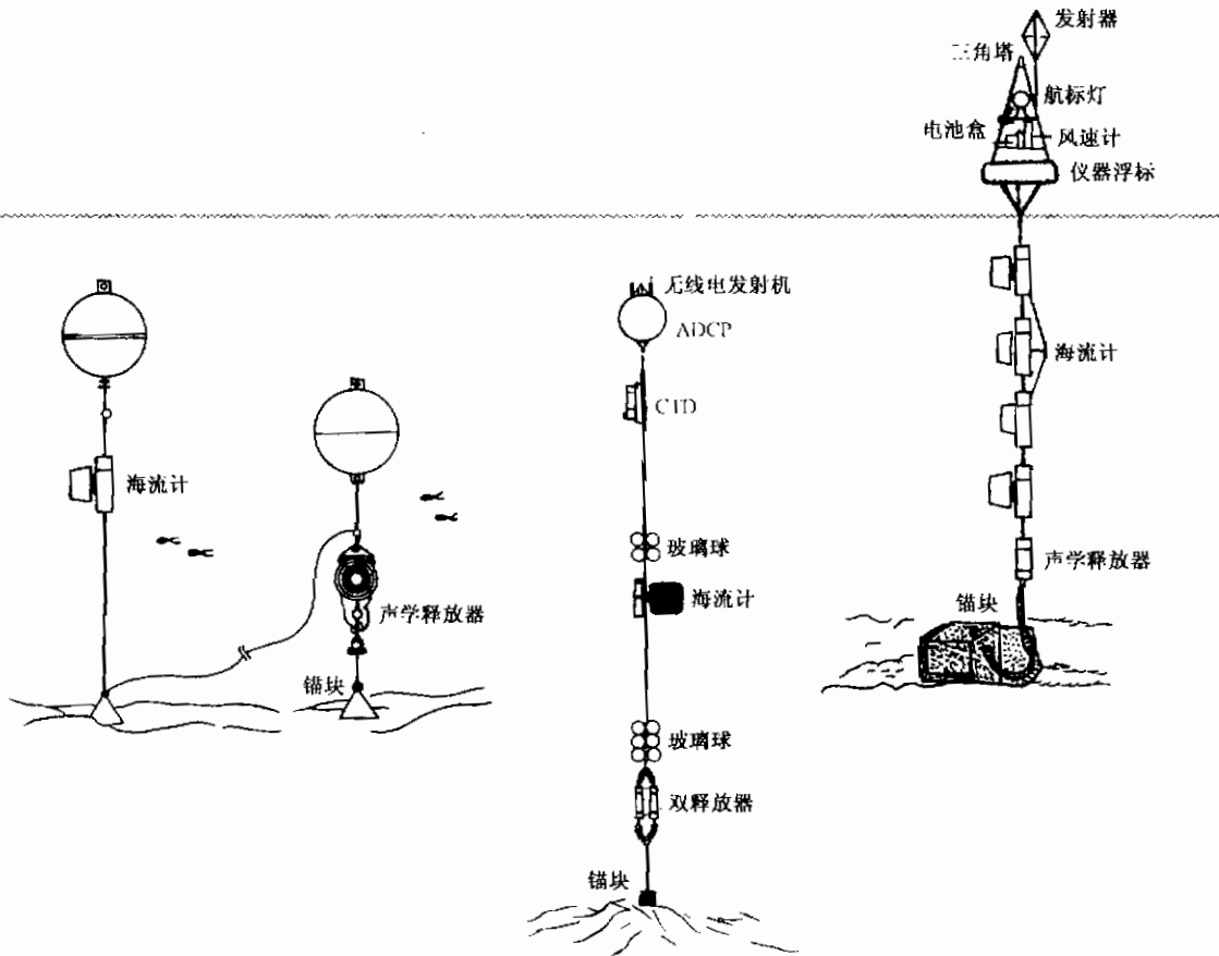
图 1 锚碇浅水应用型潜标
