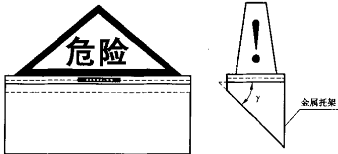
图 3 C 型标志灯
